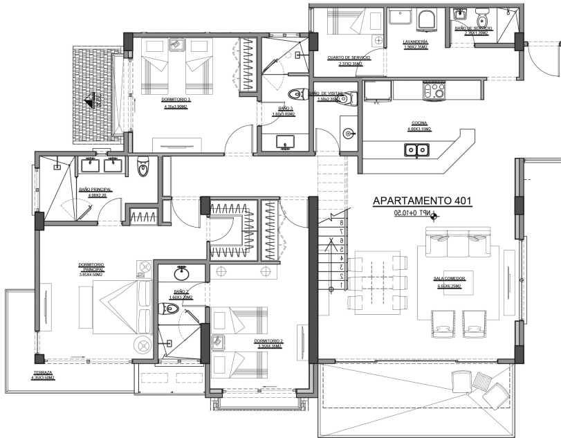
Planta Baja
